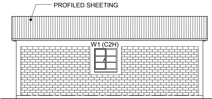
ELEVATION 3
