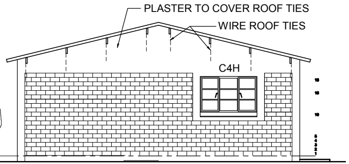
ELEVATION 2
