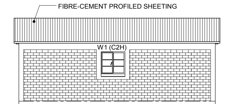
ELEVATION 3
