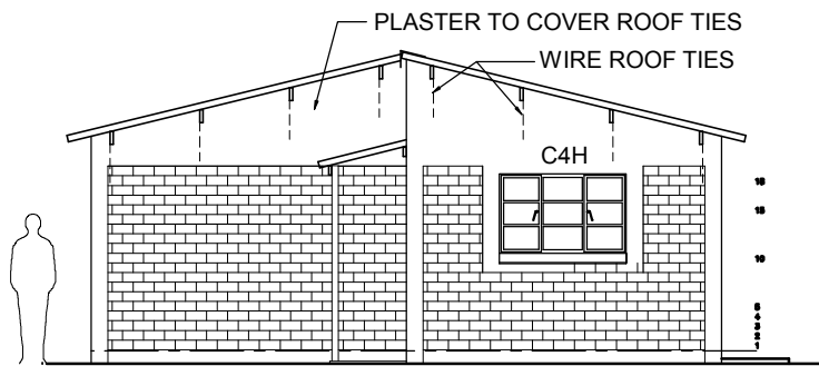
ELEVATION 2
