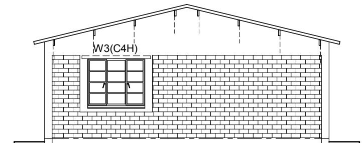
ELEVATION 4
