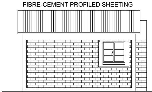
ELEVATION 3
