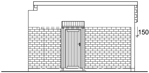
ELEVATION 1
