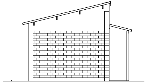
ELEVATION 4
